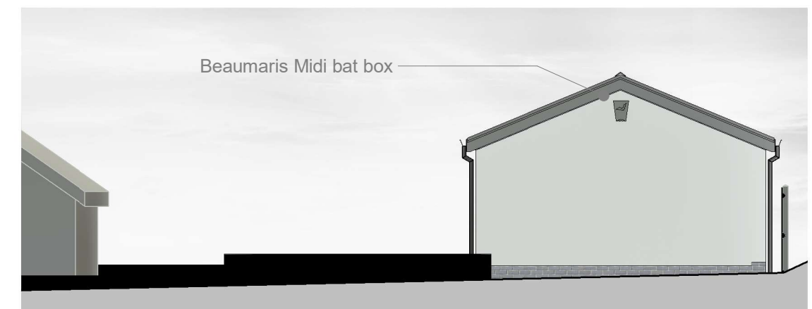
1 : 100 RIGHT ELEVATION
