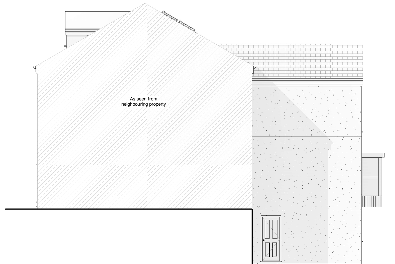
Right Elevation 1 : 100
