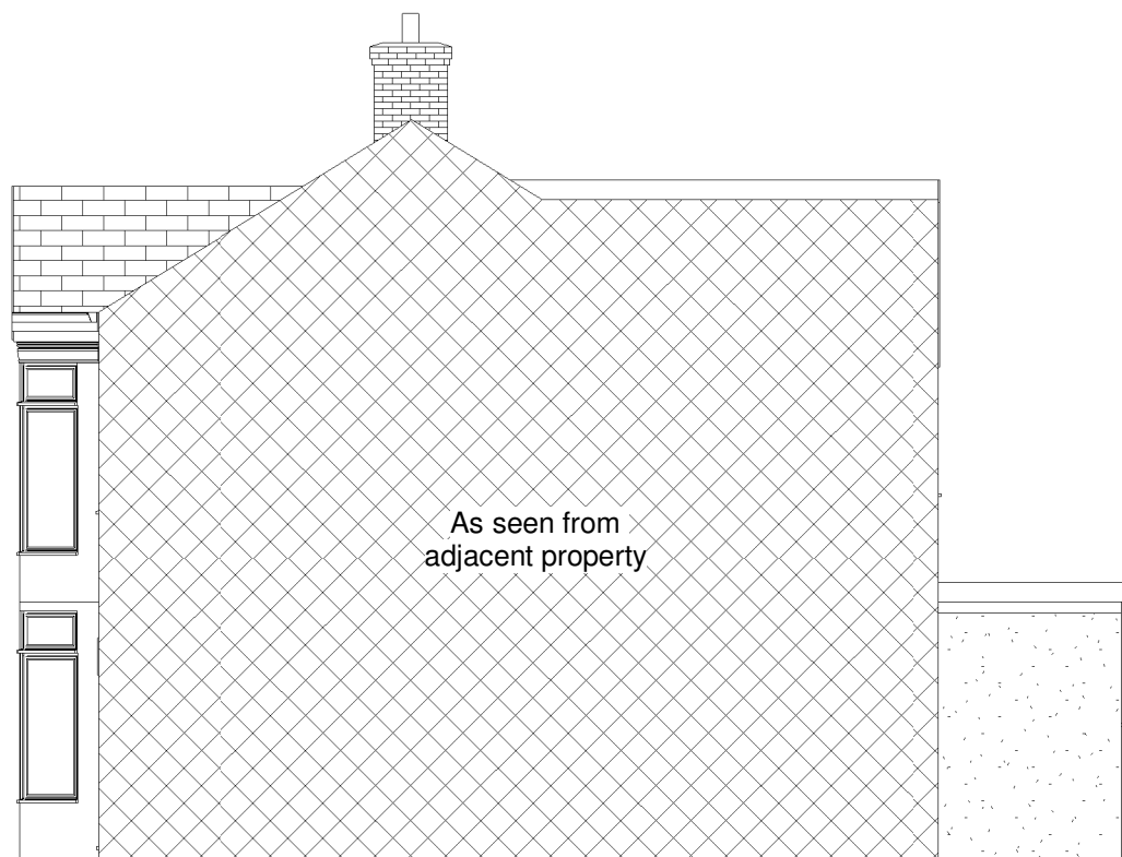
Right Elevation 1 : 100
