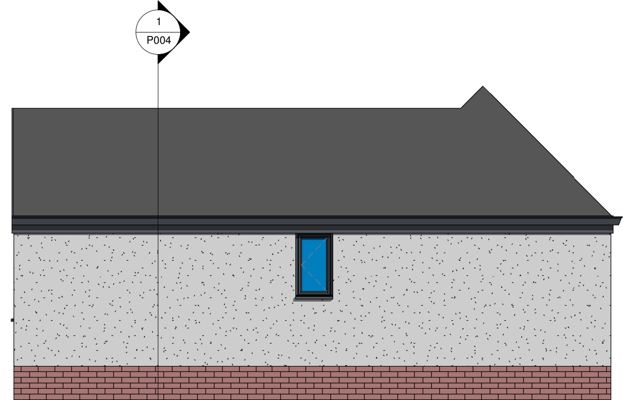
3 Right Elevation 1 : 50
