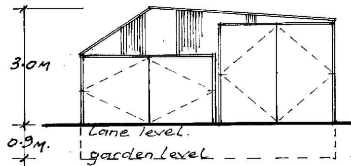
ELEVATION A
