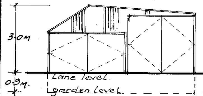
ELEVATION A
