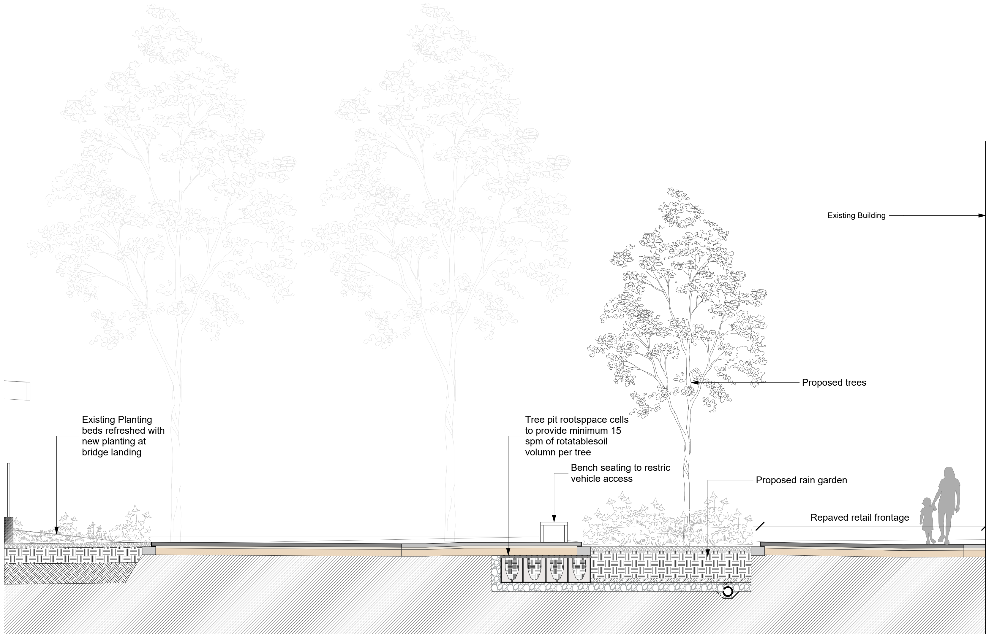
2 Section GG Scale: 1:50
