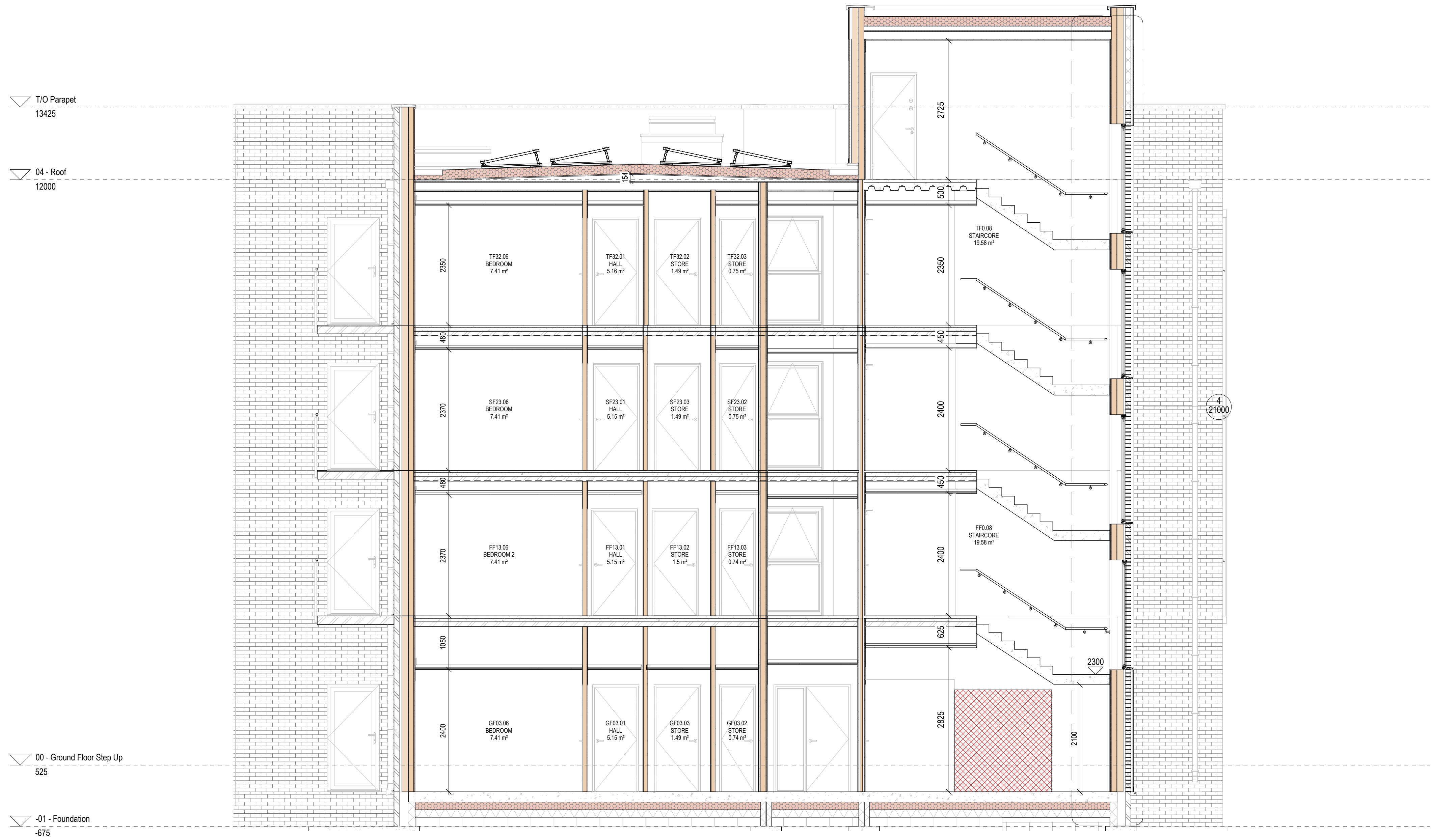
Section C Scale: 1 : 50
