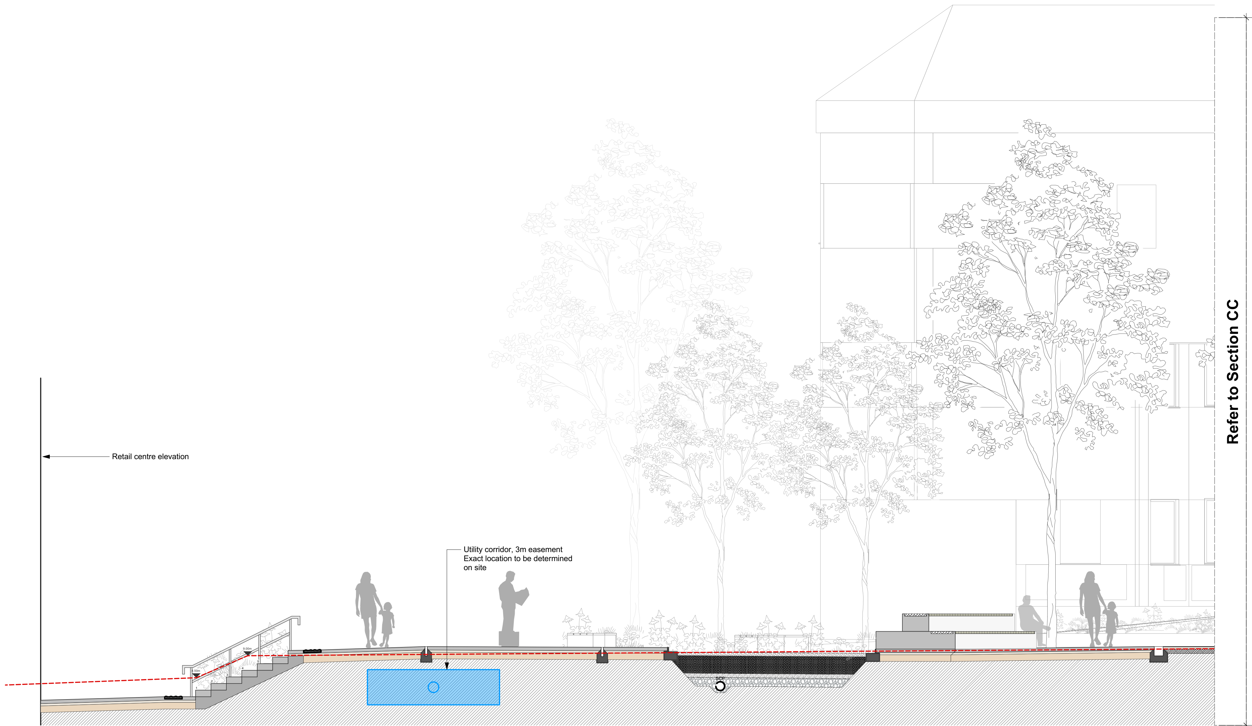
1 Section BB Scale: 1:50
