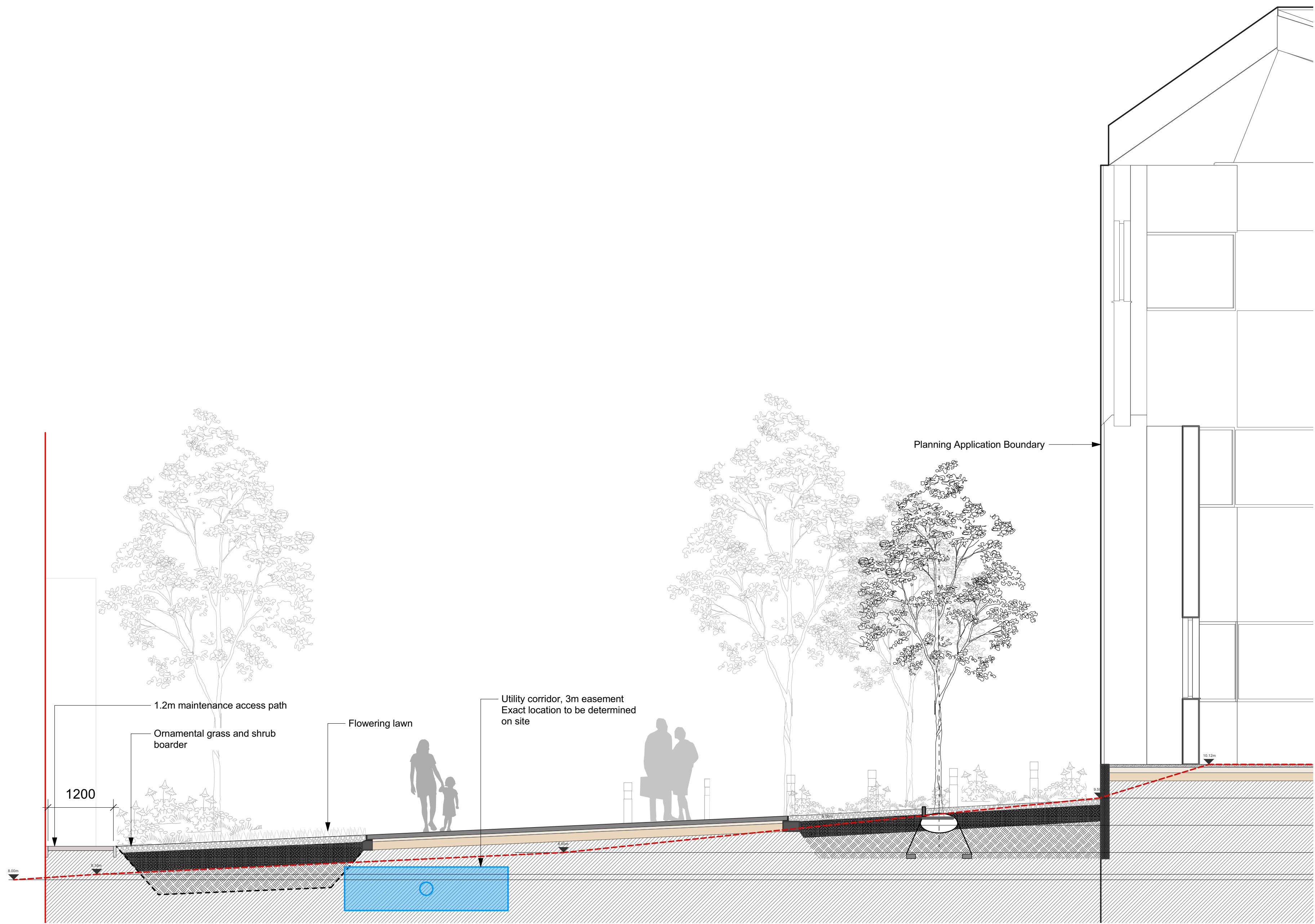
1 Section AA Scale: 1:50
