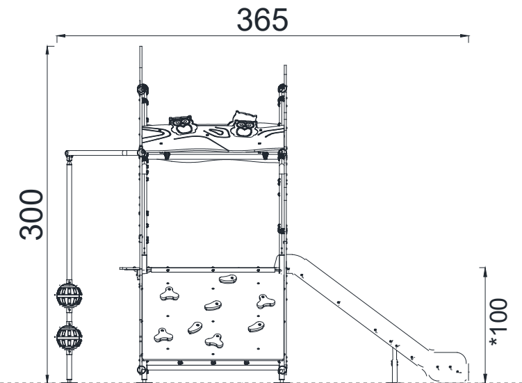
YAN GÖRÜNÜŞ / SIDE VIEW
