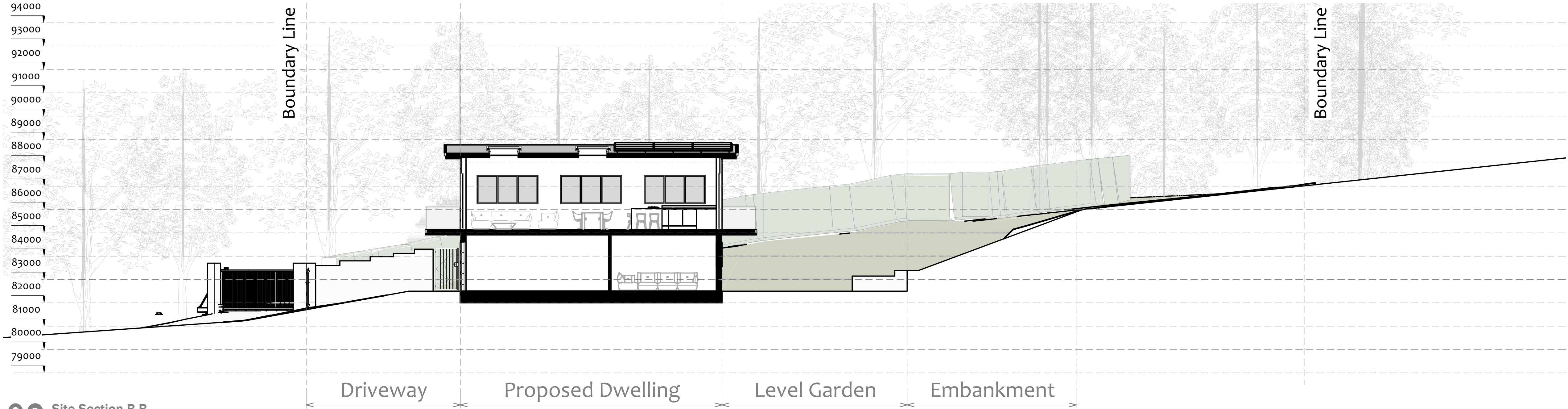
02 Site Section B-B 1 : 100
