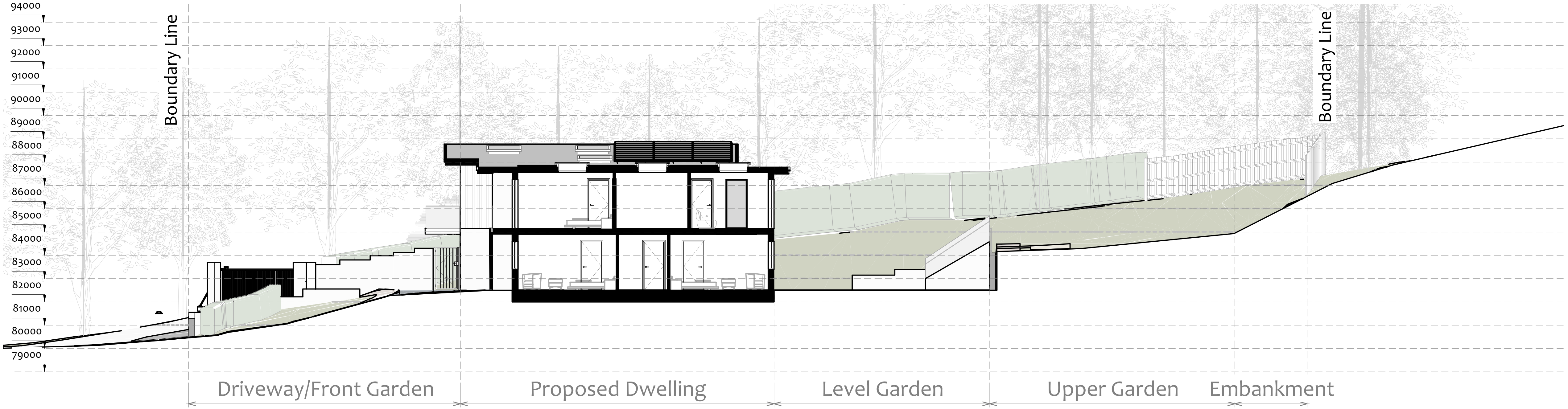
01 Site Section A-A 1 : 100
