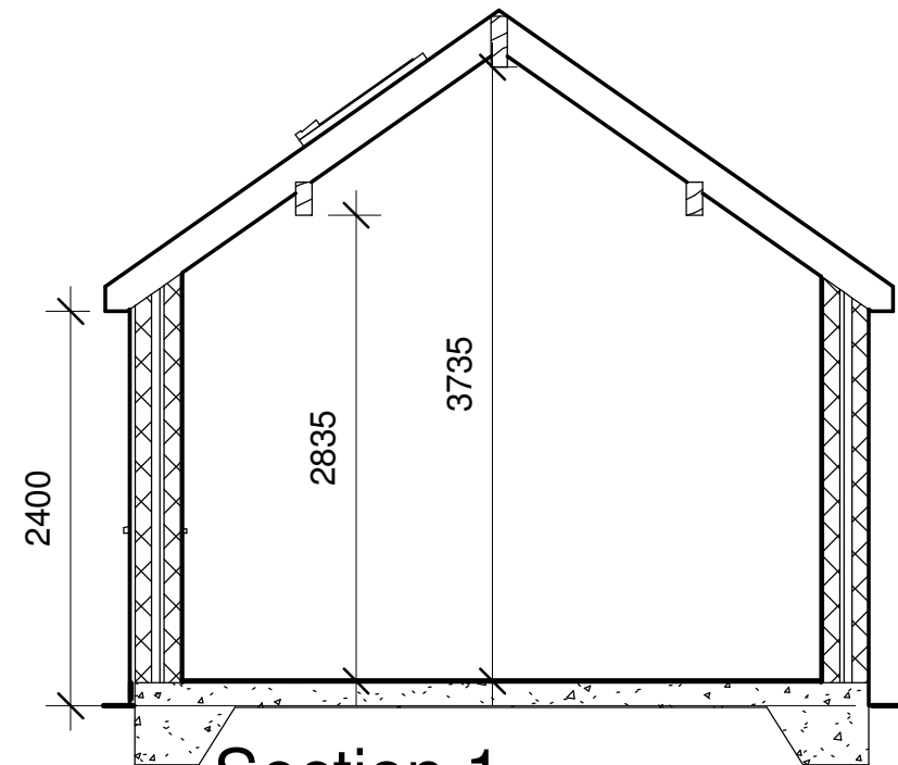
6 Section 1 1 : 50
