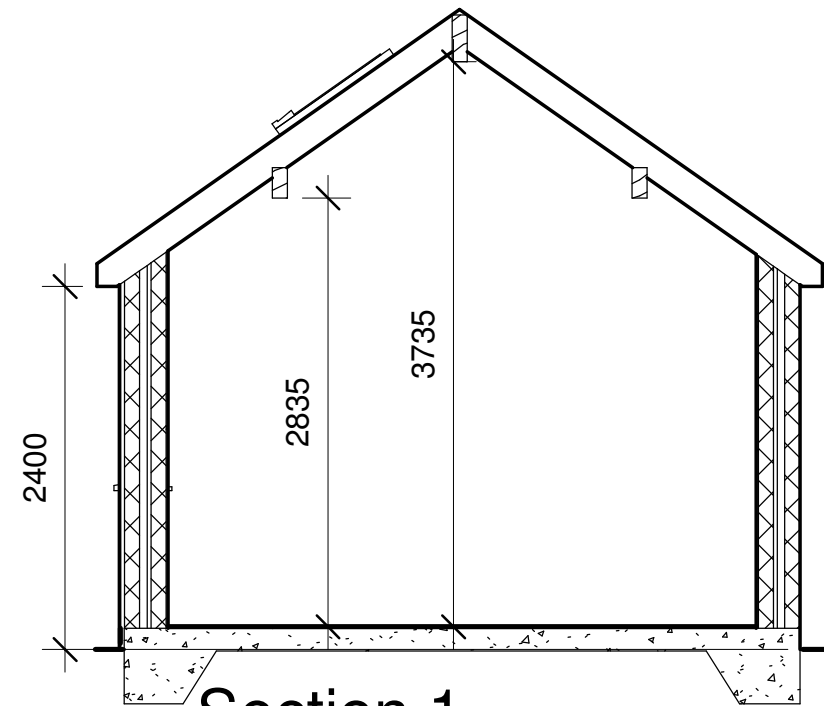
6 Section 1 1 : 50
