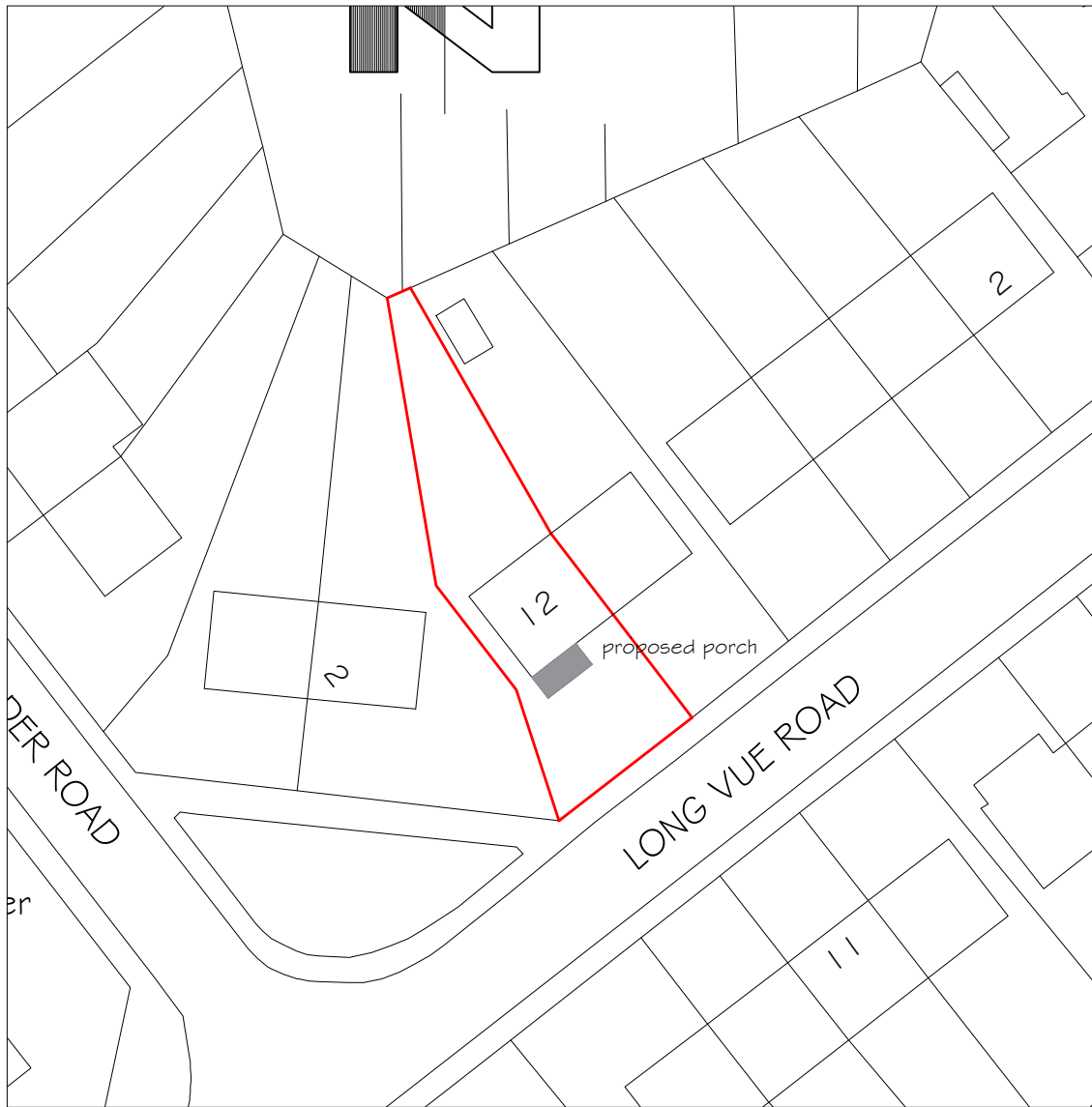
SITE PLAN 1:500
