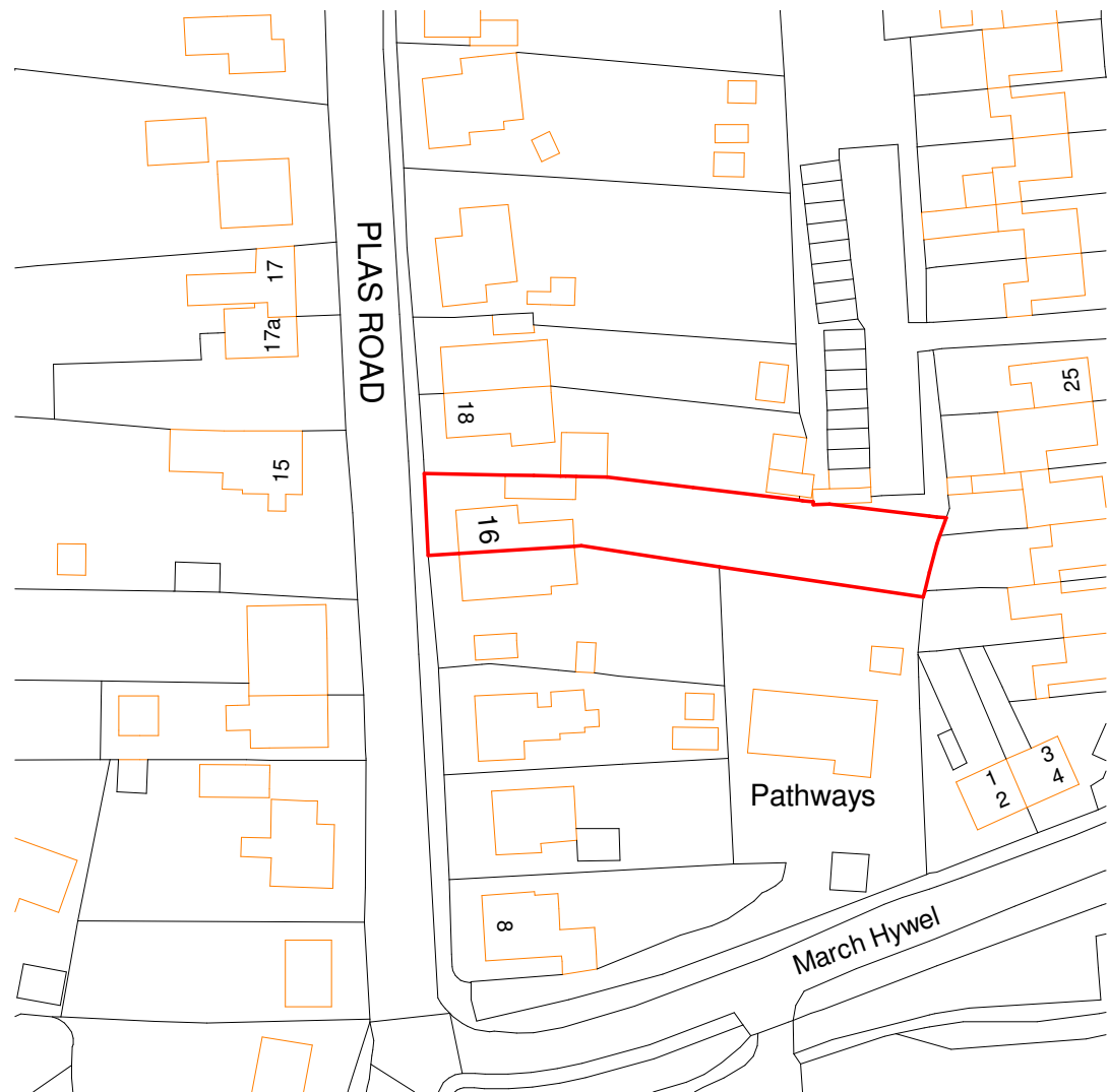
2 Existing Site Plan 1 : 1000
