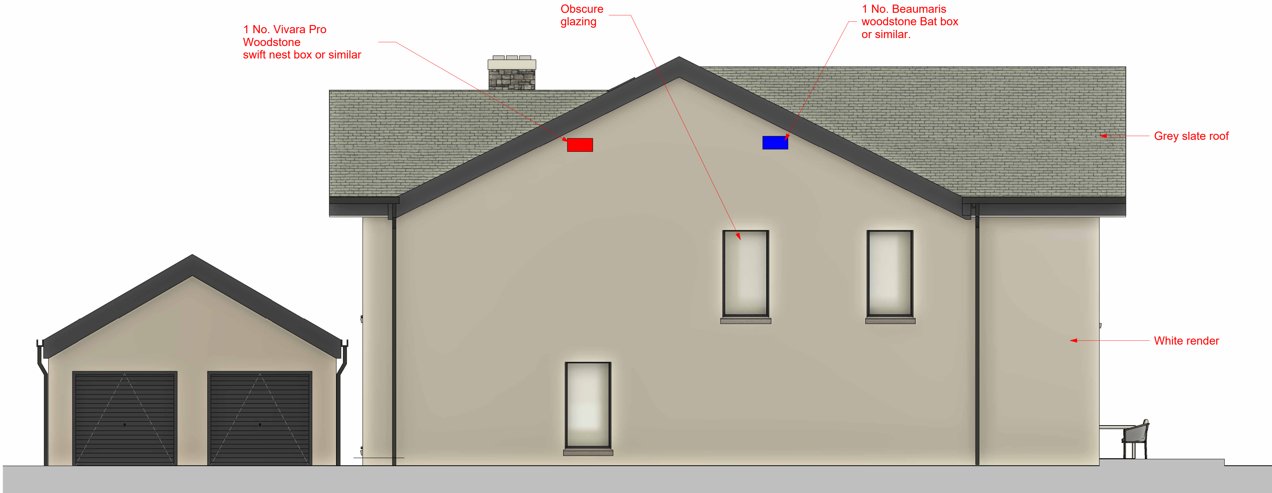
East 1 : 50
