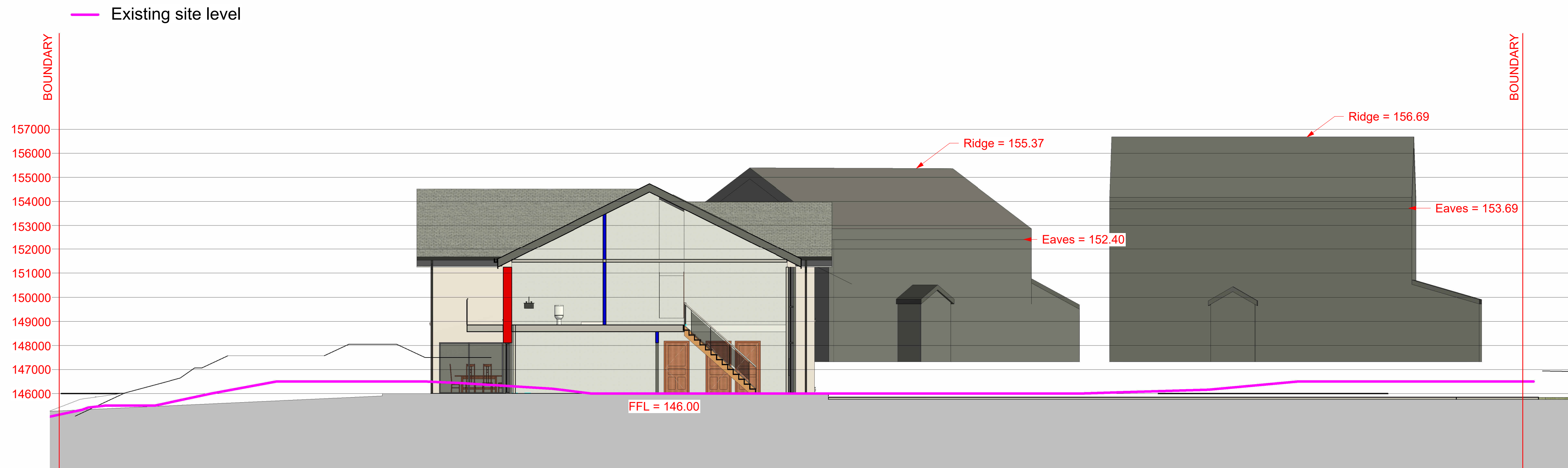
1 Section AA 1 : 100
