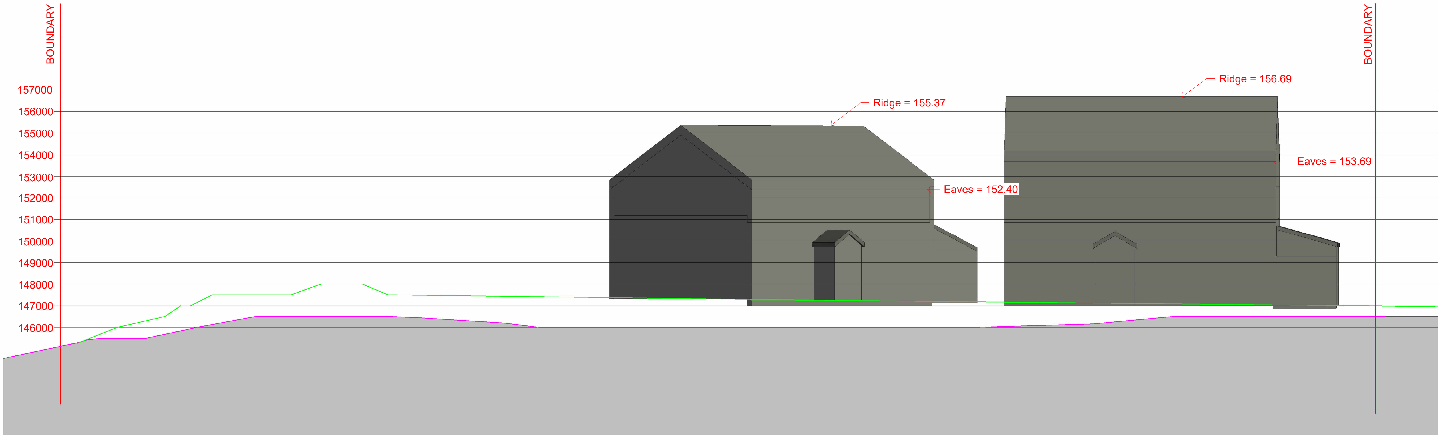
1 Section AA 1 : 100
