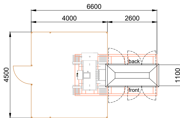
TOP ELEVATION
