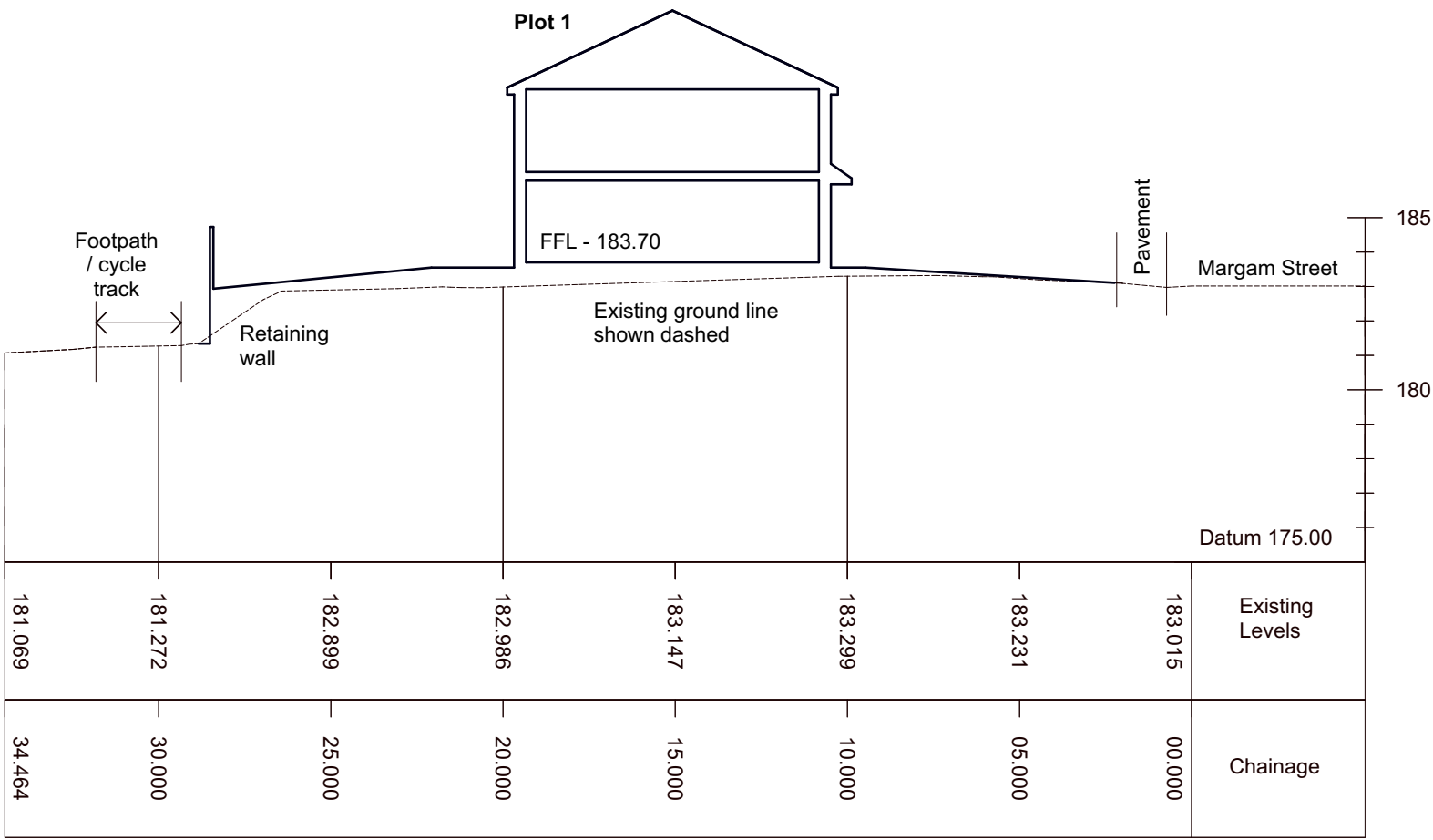
Section A-A
