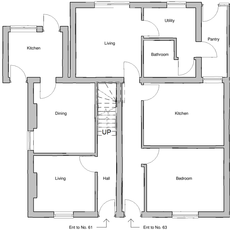
Existing GF 1 : 100
