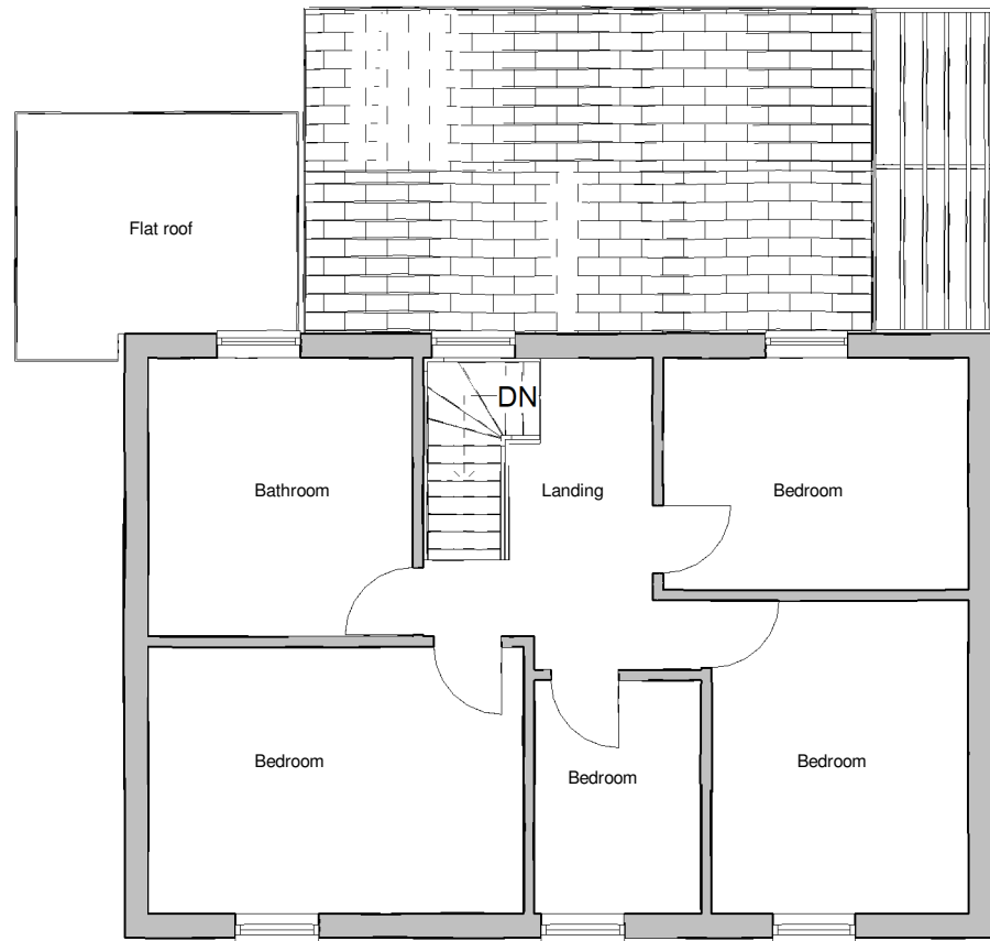
Existing FF 1 : 100
