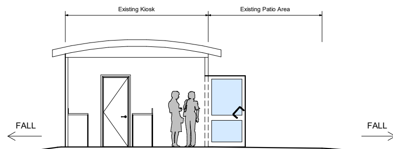
Existing Section A-A 1 : 50
