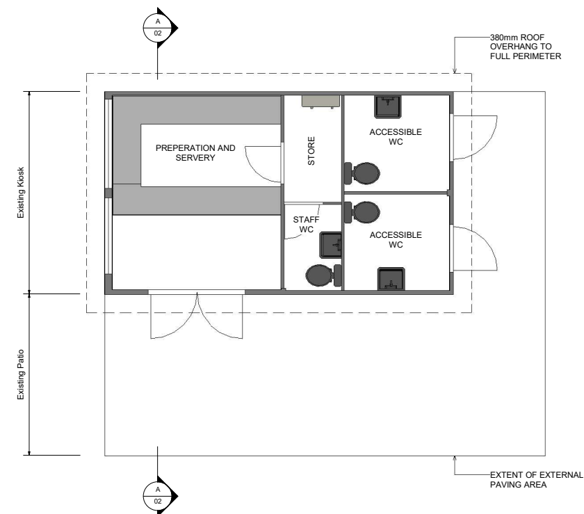
Kiosk Existing Plan 1 : 50
