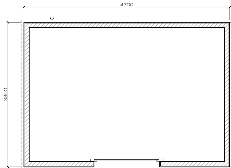
PLAN 1 : 50
