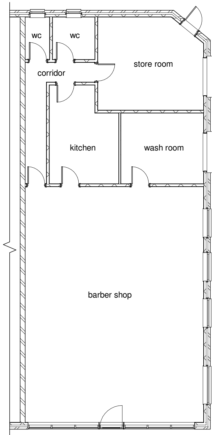
Existing GF 1 : 100
