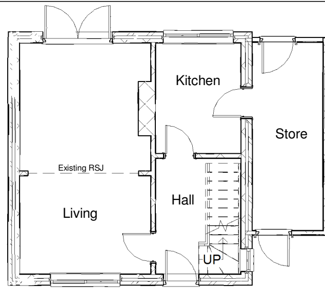
Existing GF 1 : 100
