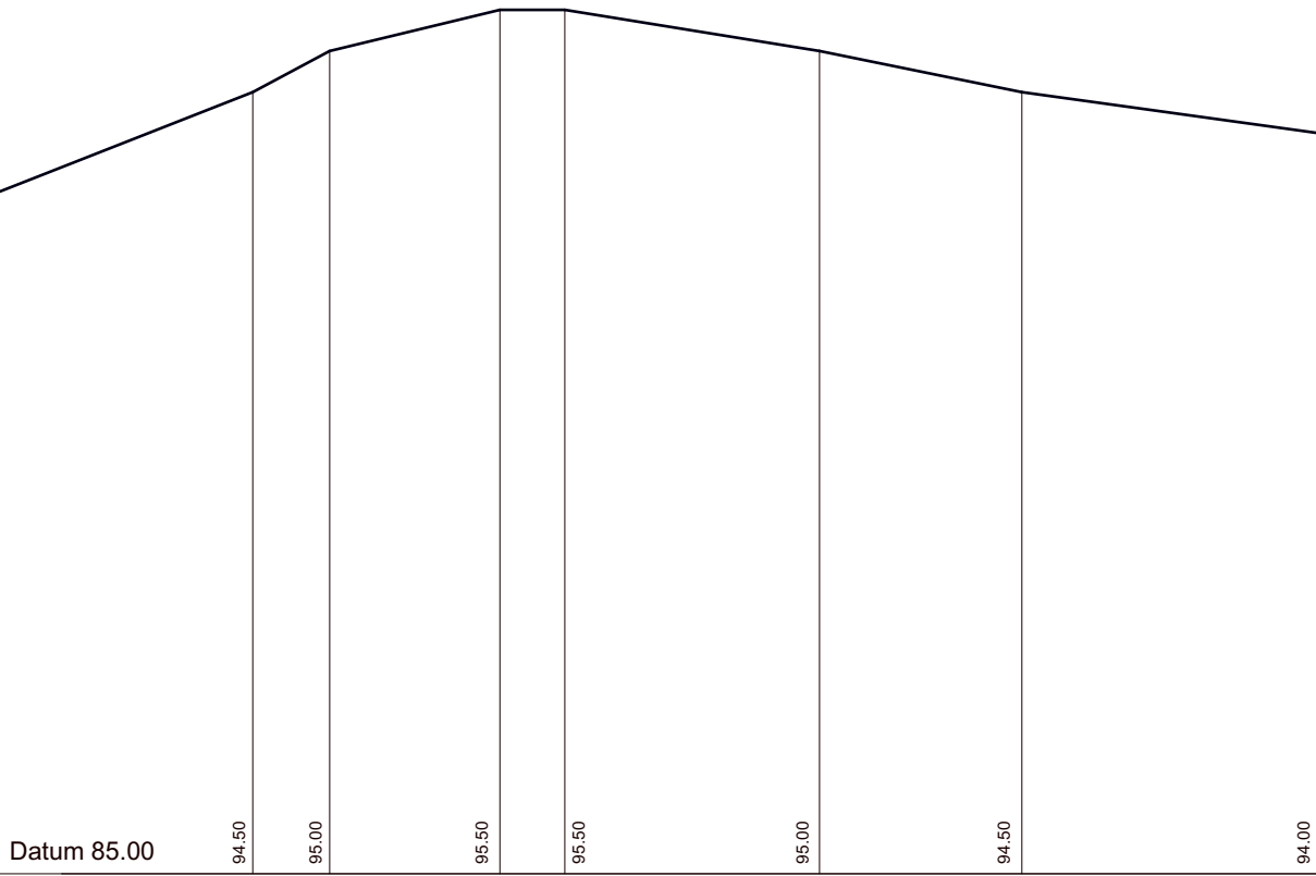
Site Section D-D
