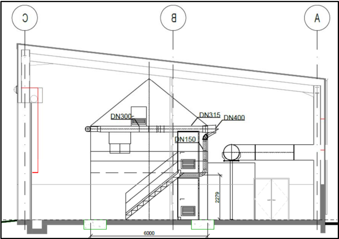
Right Elevation
