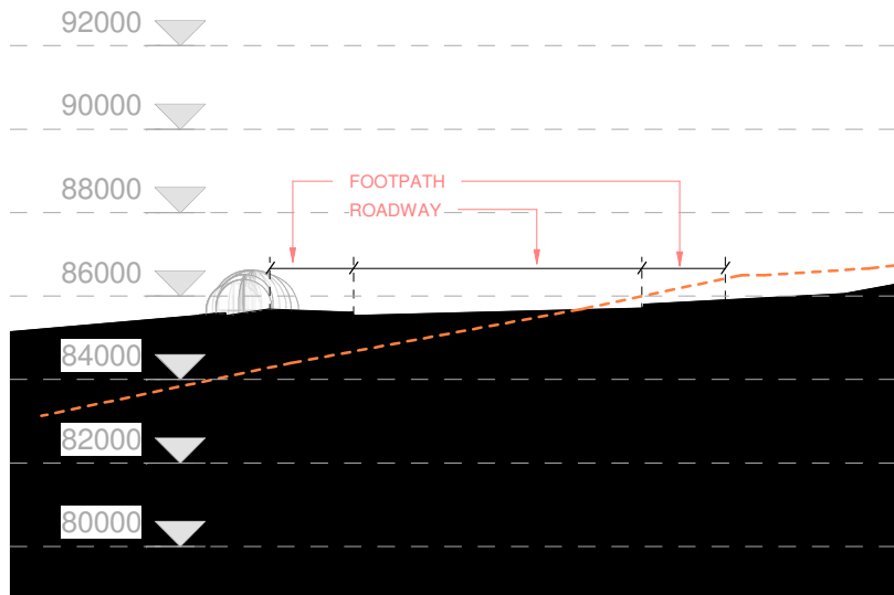
ROAD SECTION 4 1 : 200
