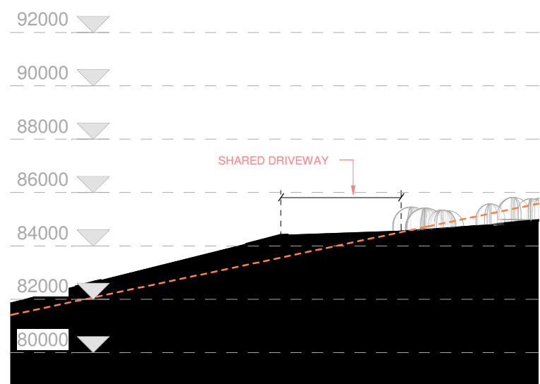
ROAD SECTION 7 1 : 200
