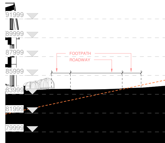
ROAD SECTION 6 1 : 200
