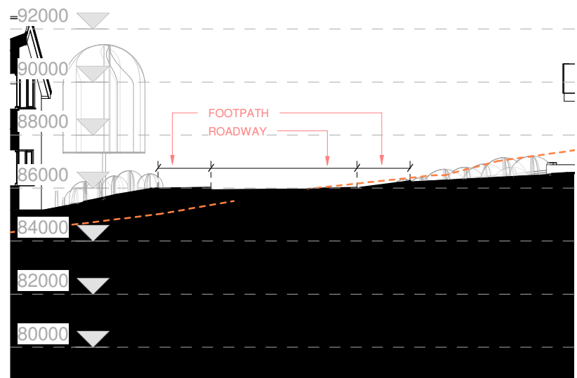
ROAD SECTION 3 1 : 200
