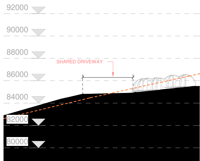
ROAD SECTION 9 1 : 200
