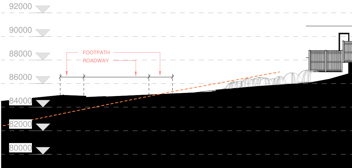
ROAD SECTION 5 1 : 200
