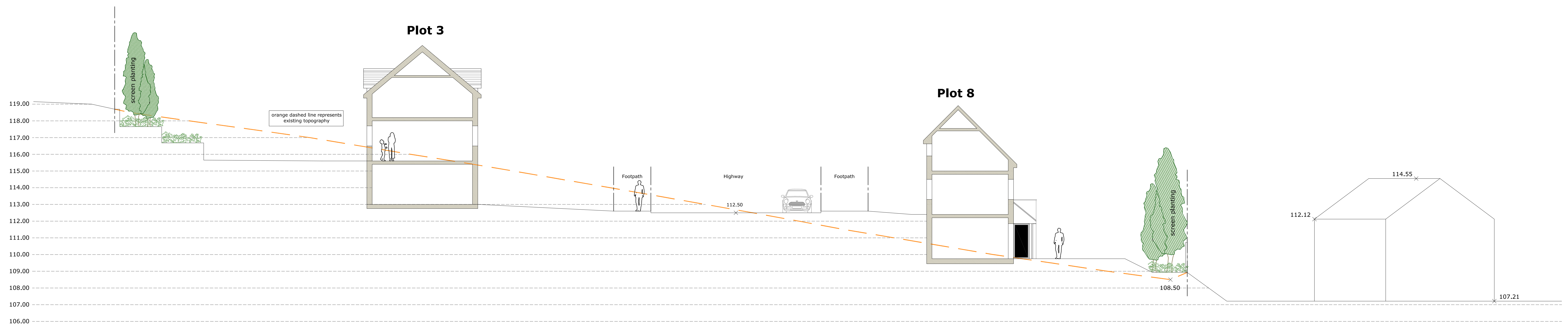
Site section B-B
