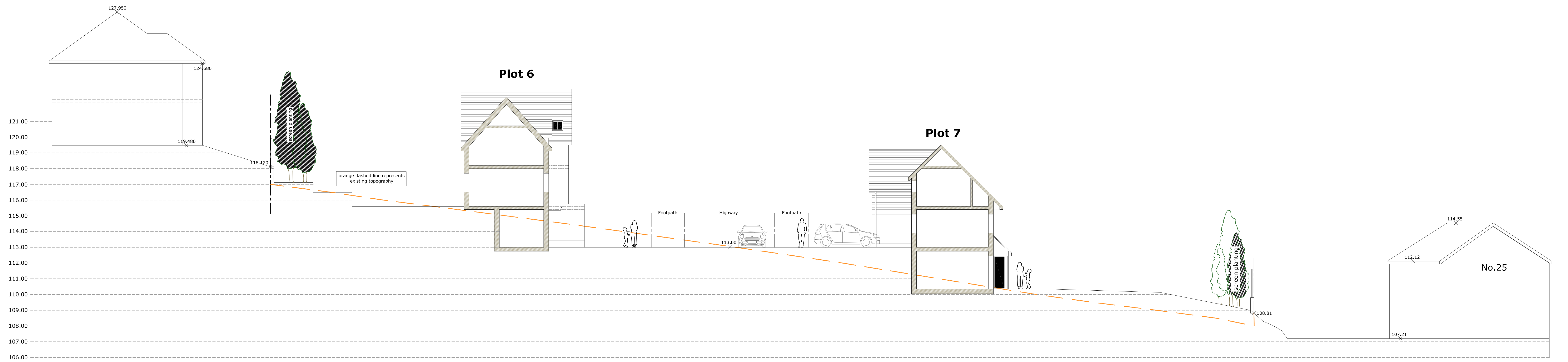
Site section A-A
