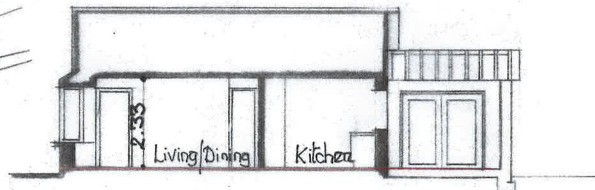
Section A-A
