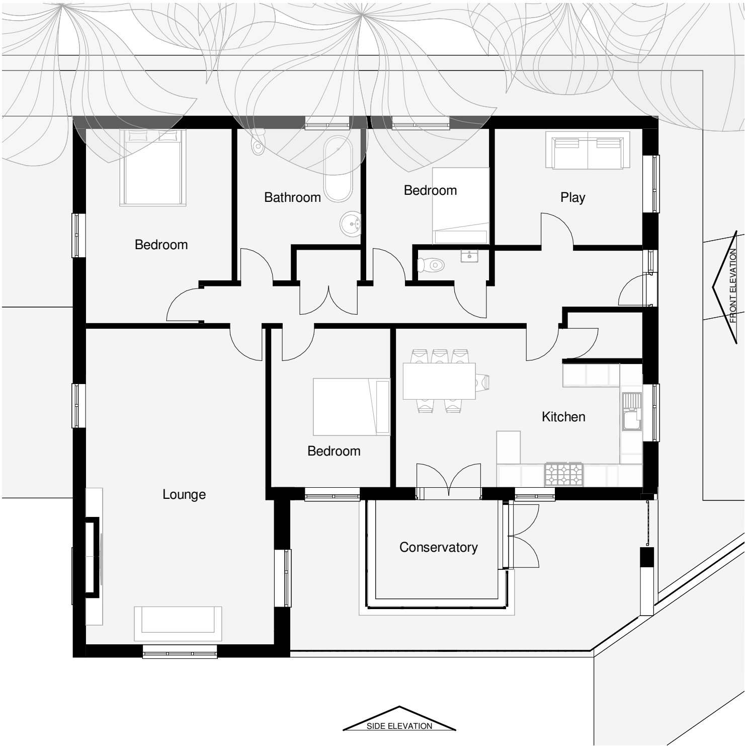
GFL - EXISTING 1 : 100
