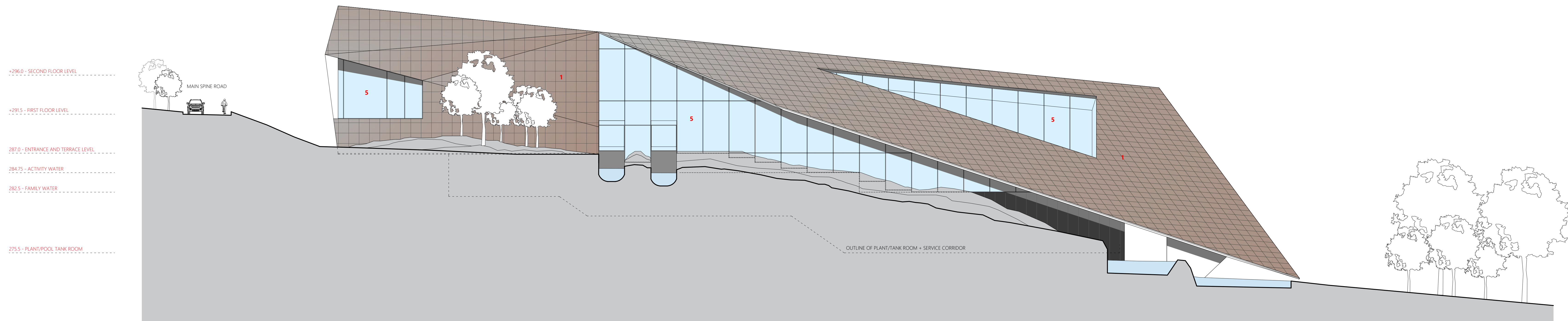
Elevation 3 1:200
