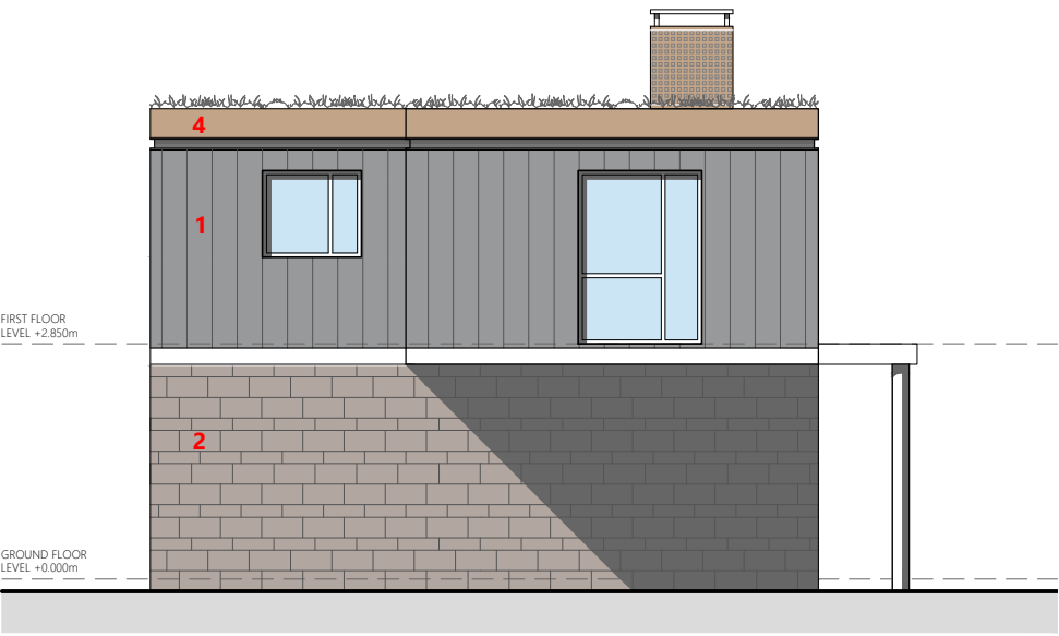
Elevation A
