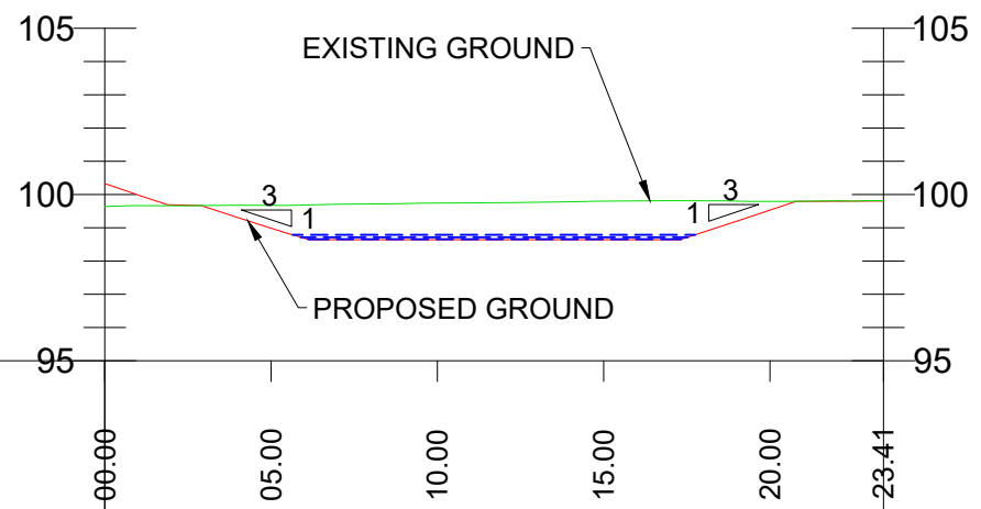
SECTION A-A SCALE: H 1:200,V 1:200 DATUM: 95.000
