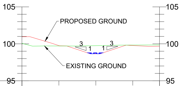
SECTION B-B SCALE: H 1:200,V 1:200 DATUM: 95.000
