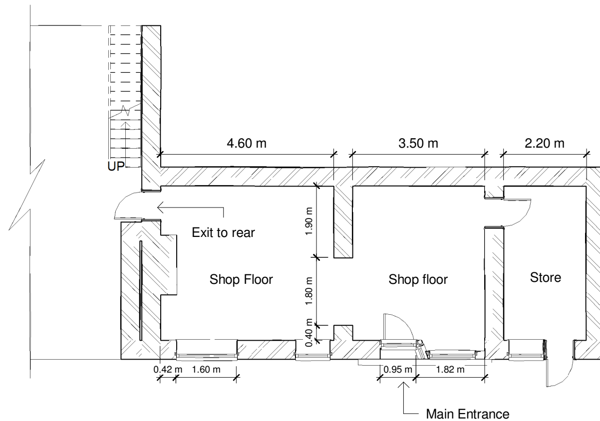
Existing GF 1 : 100
