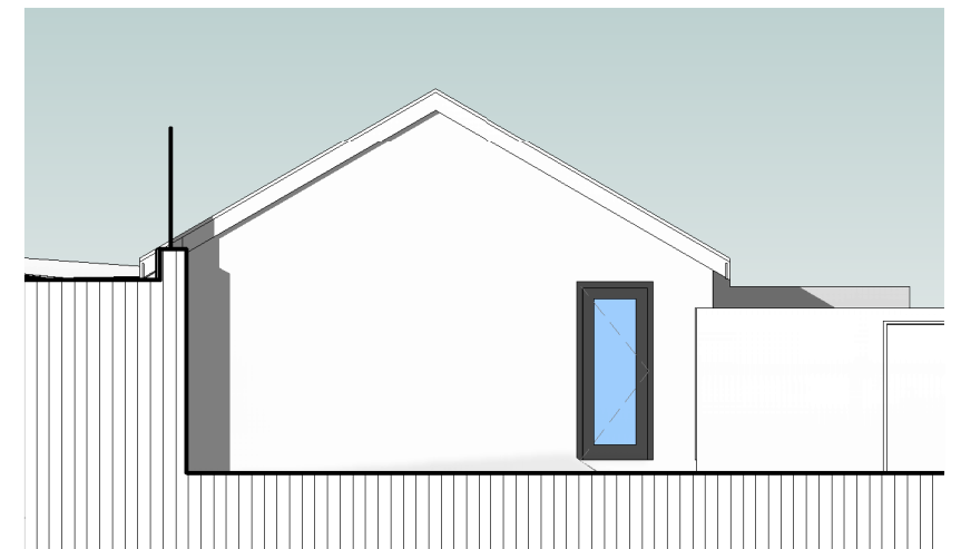
GARAGE ELEVATION 04 1 : 100
