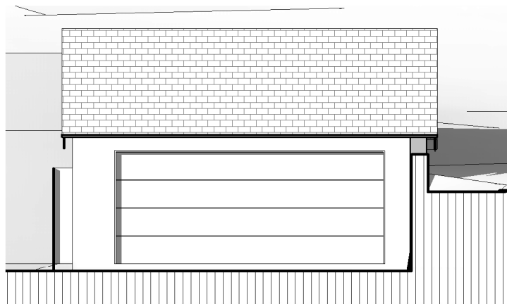
GARAGE ELEVATION 01 1 : 100
