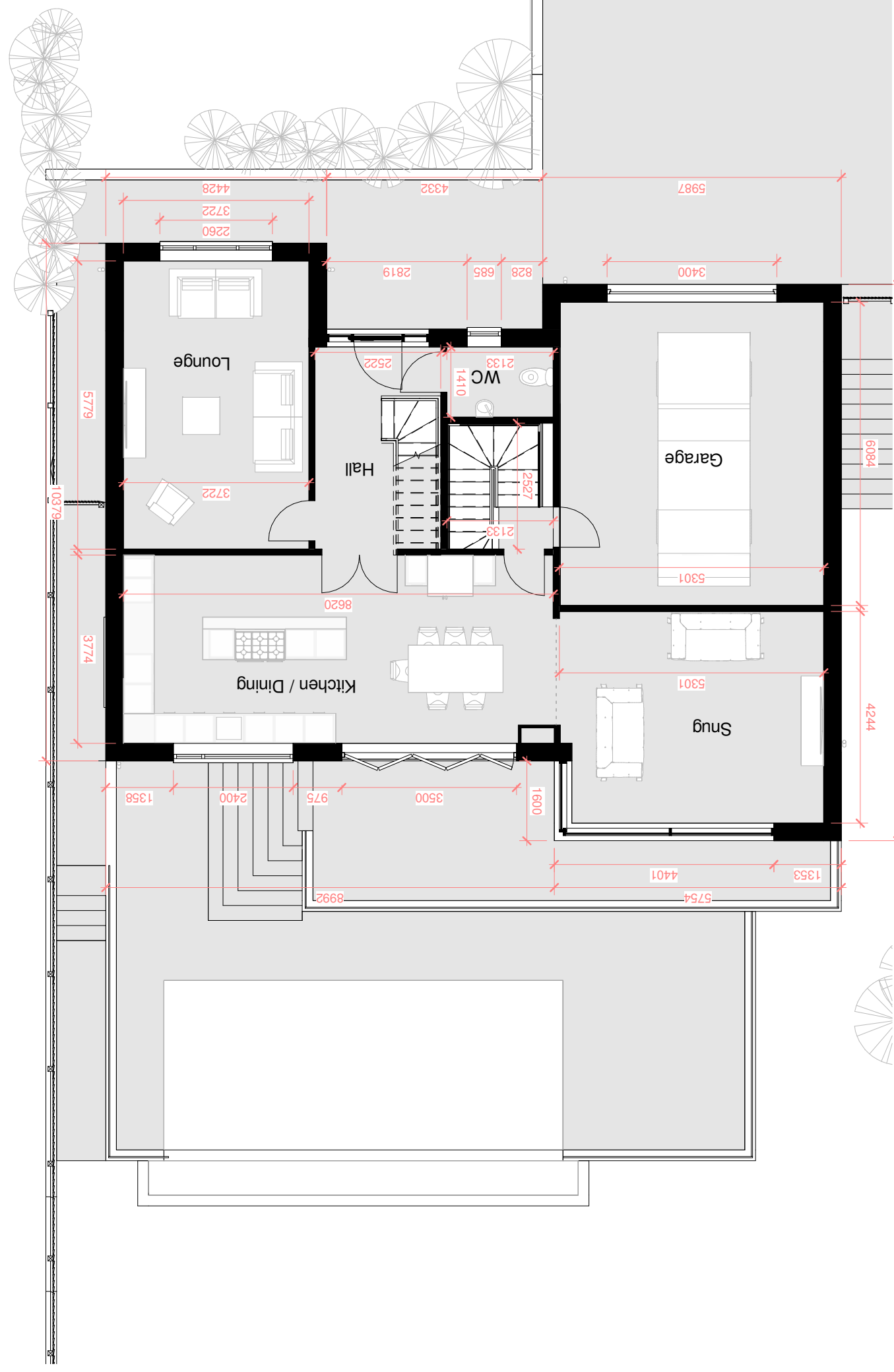
PLOT 3 - GFL 1 : 100
