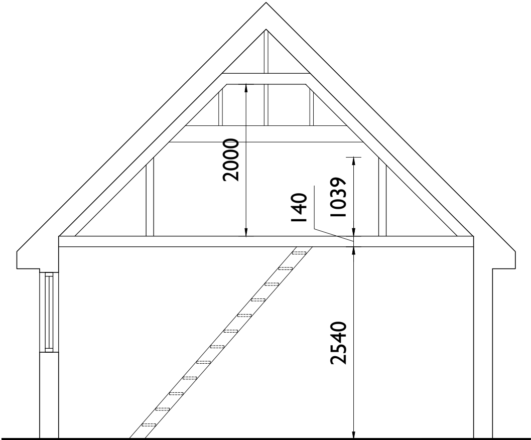
Section A-A 1:50
