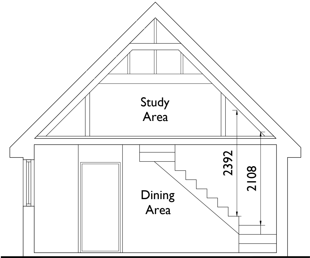
Section A-A 1:50
