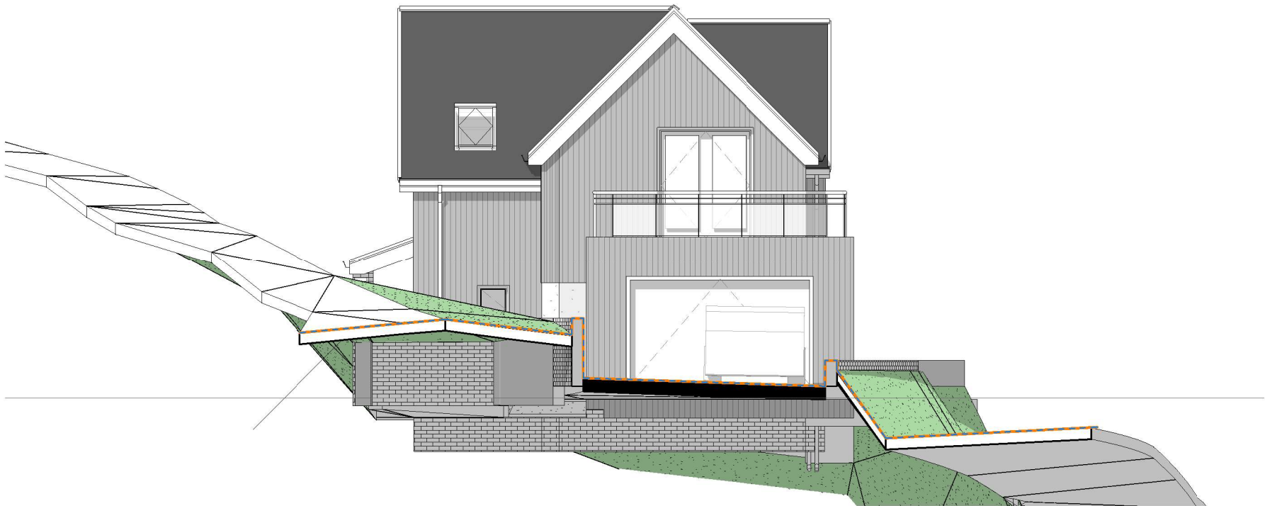
SECTION S1 1 : 100
