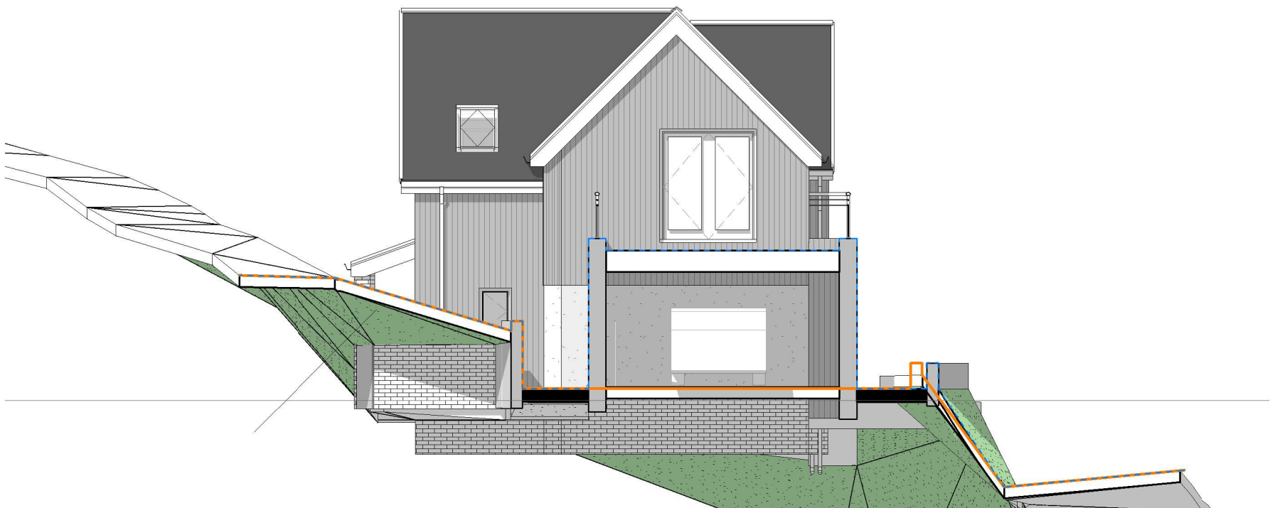
SECTION S2 1 : 100
