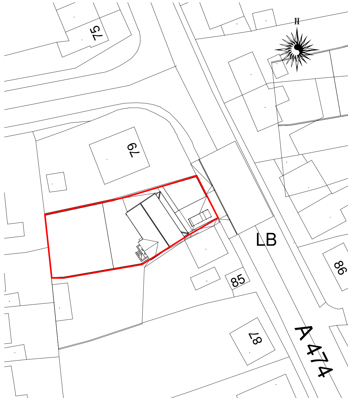
BLOCK PLAN 1 : 500
