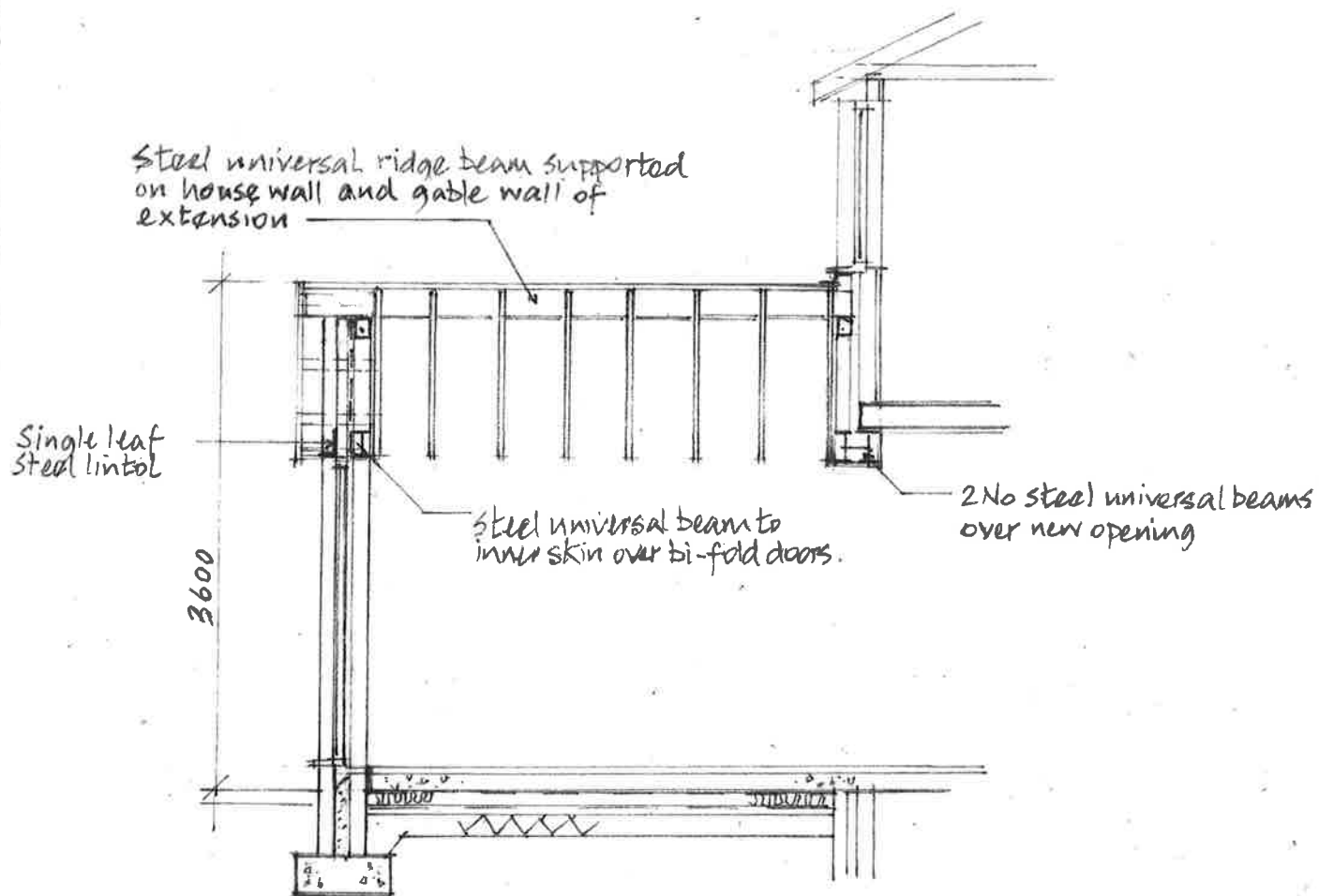
Section A-A (1:50).
