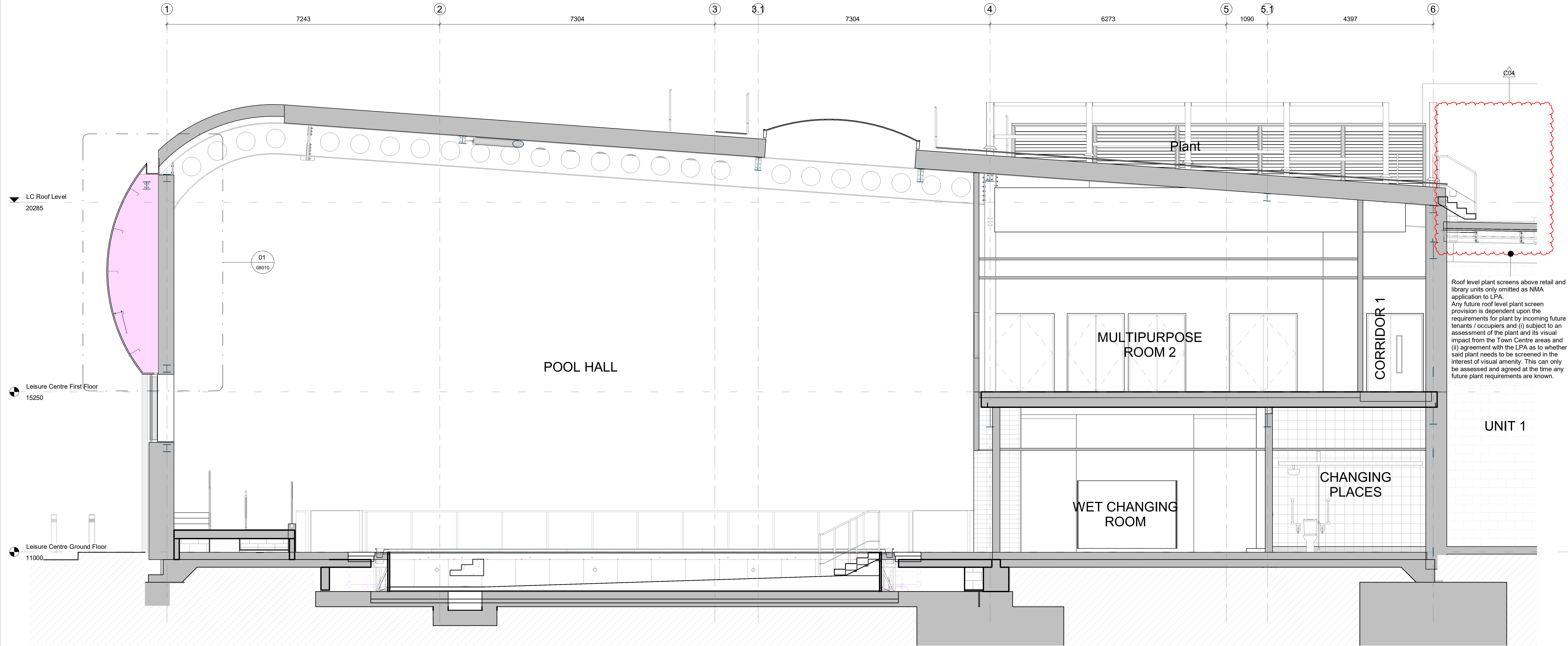
Section C 1 : 50
