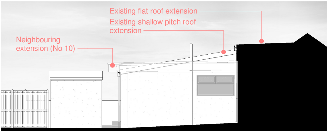
EXISTING LEFT 1 : 100
