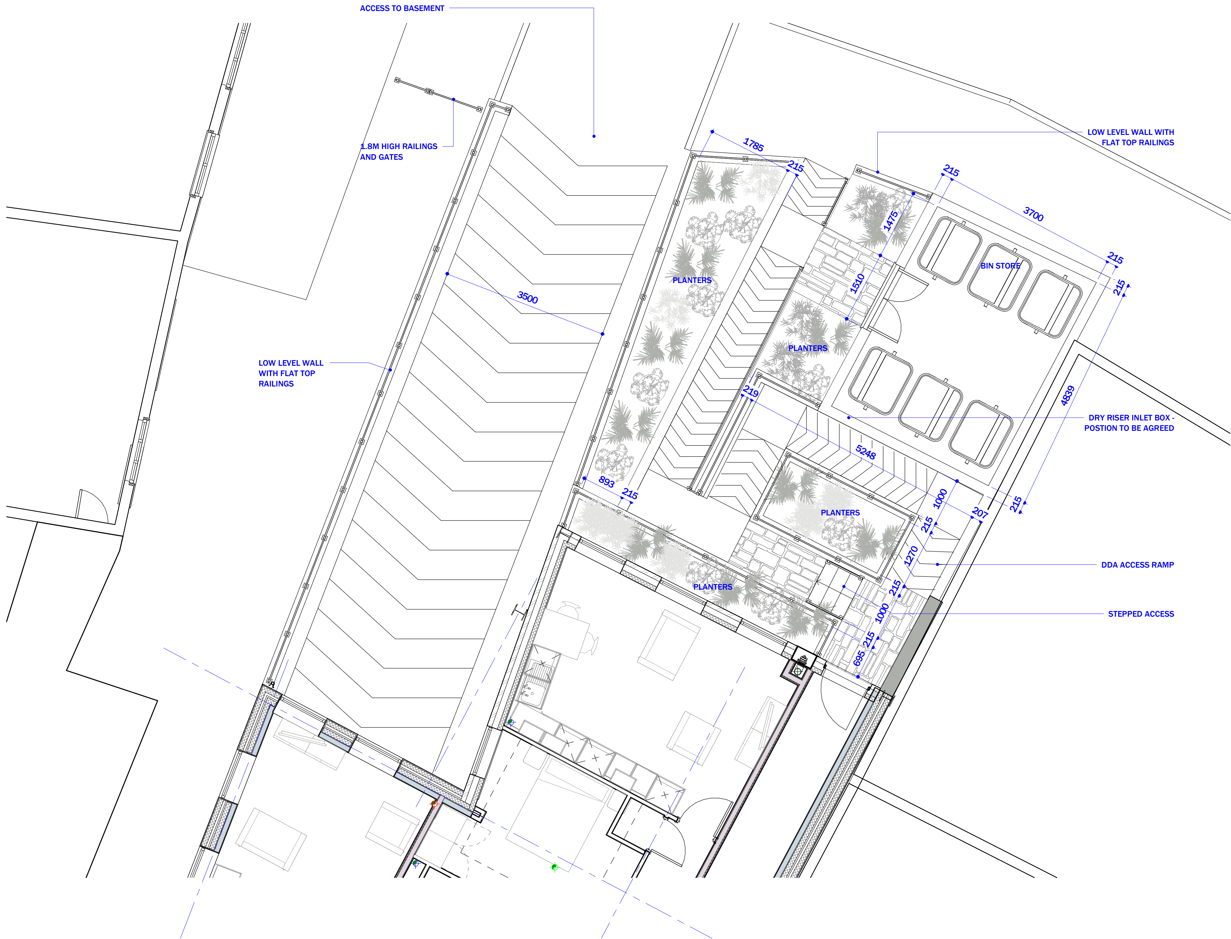
01 SITE ENTRANCE/BIN STORE LAYOUT 1 : 50
