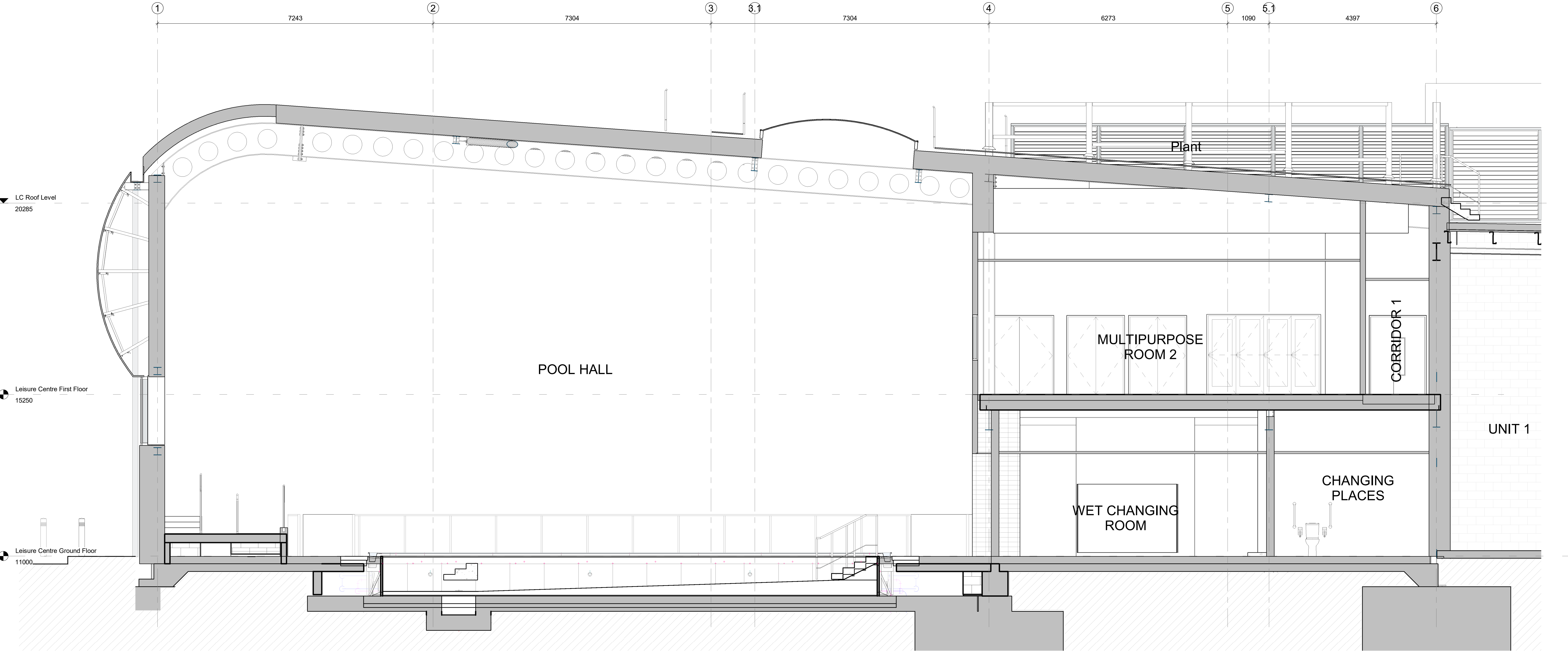
Section C 1 : 50
