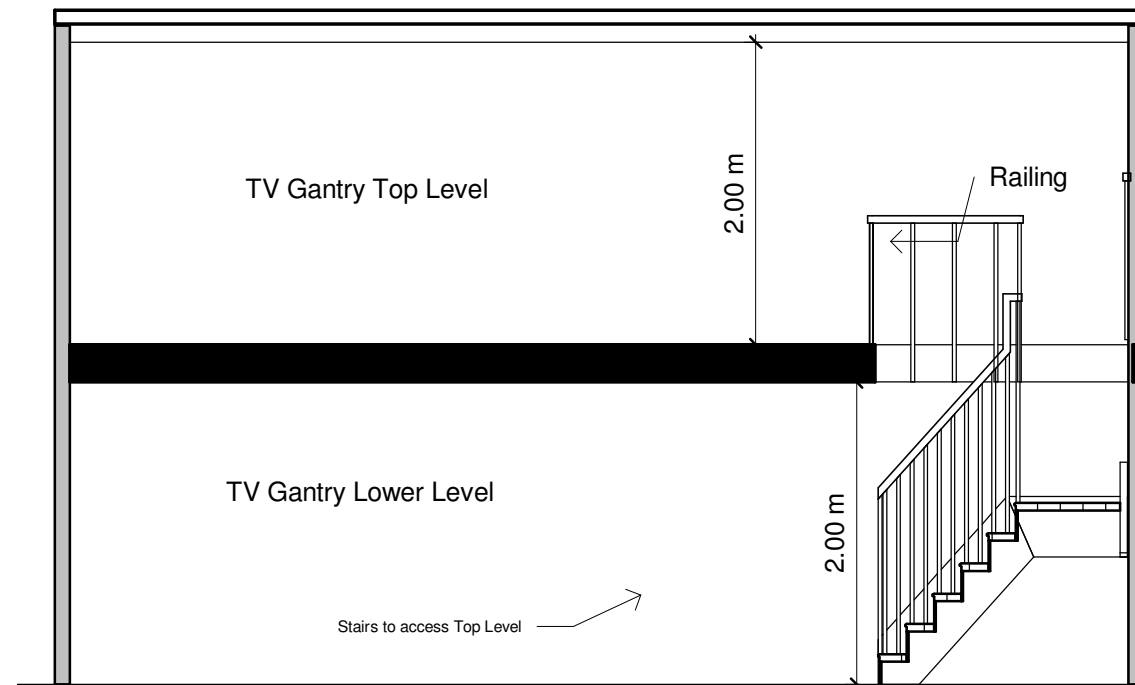
1 Section 1 A-A 1 : 50
