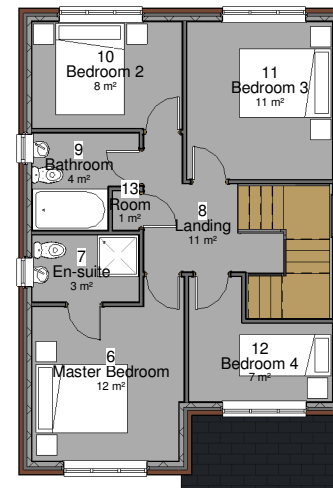
3 Plot 1 - FF 1 : 100
