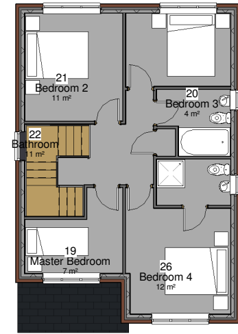
4 Plot 2 - FF 1 : 100
