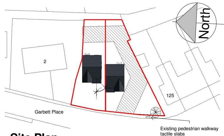
2 Site Plan 1 : 500
